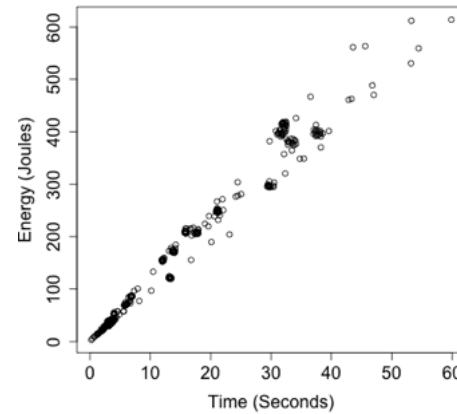
(b) AProVE
